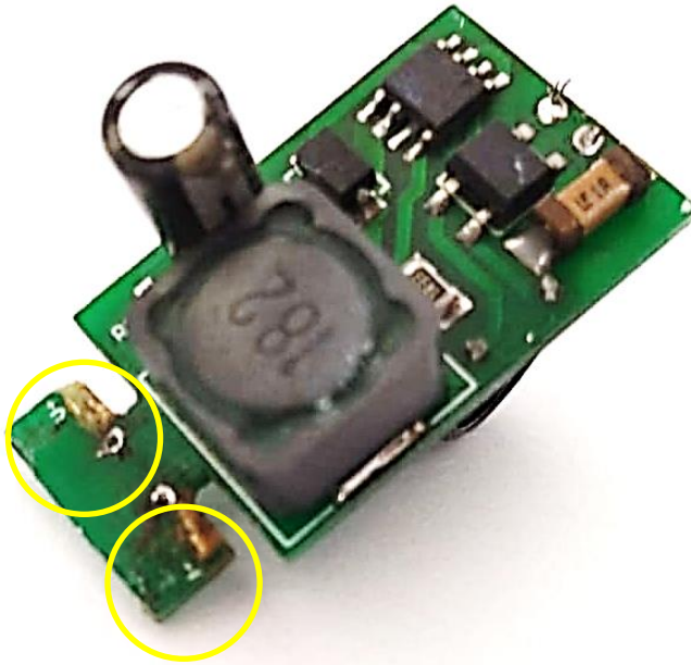
Figura 5. Vista superior de la tarjeta electrónica del conversor posterior a la prueba
