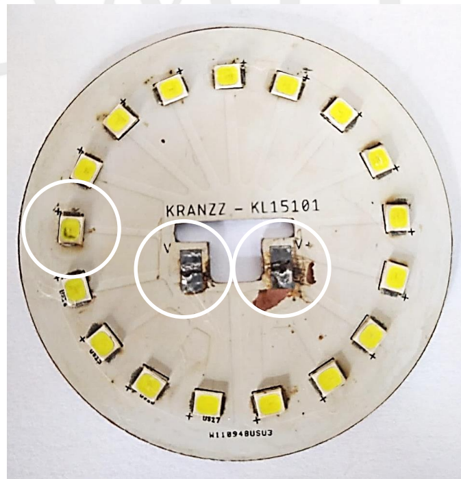
Figura 4. Tarjeta de chips LED luego de la segunda prueba
