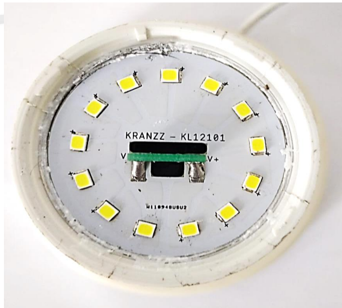
Figura 6. Vista superior de la tarjeta de chips LED después de la prueba
