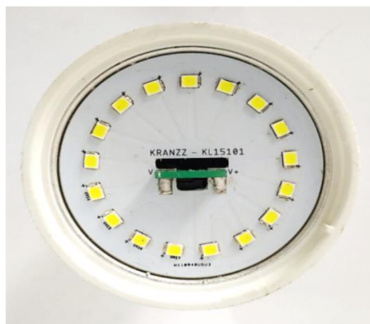
Figura 2. Vista superior durante el ensamblaje del foco sin pasta de transferencia térmica Kranzz
