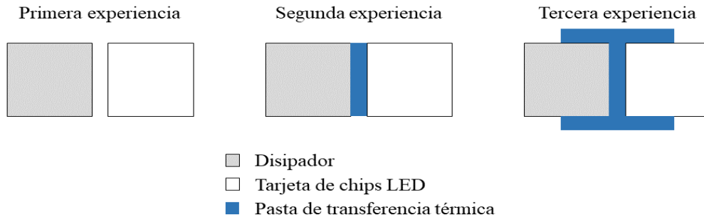
Figura 1. Esquema de la sección transversal de la unión entre disipador y tarjeta de chips LED
